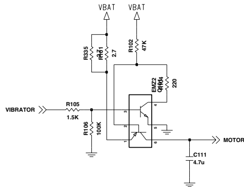
VIBRATOR_CKTs
