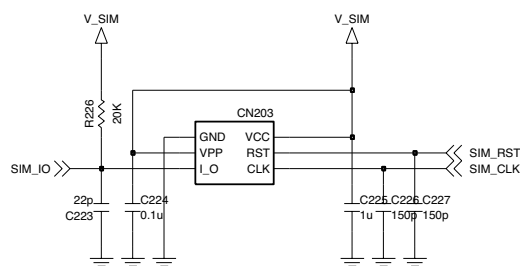
SIM I/O CKTs
